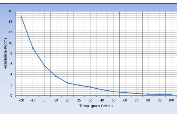
Temperatura x Resistência
